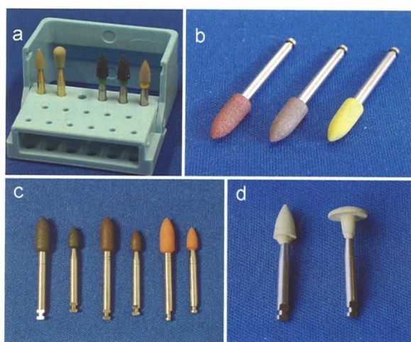
ダイヤモンドポイント。a: ジルコシャイン (松風), b: セラムダイヤモンド (モリタ) c: セラシャイン (GC), d: セラダイヤモンドスーパーファースト (Dedeco/茂久田)
