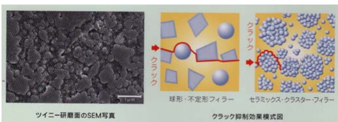
図 ツイニー研磨後のSEM写真
